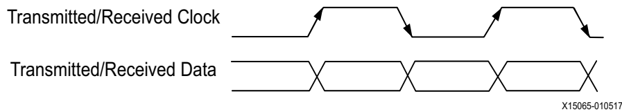
Figure 3-2: EDGE DDR
